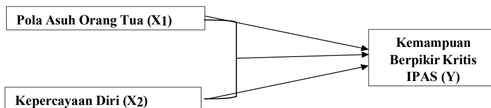
Gambar 1 Hubungan antar Variabel X 1 ,X 2 dan Y
